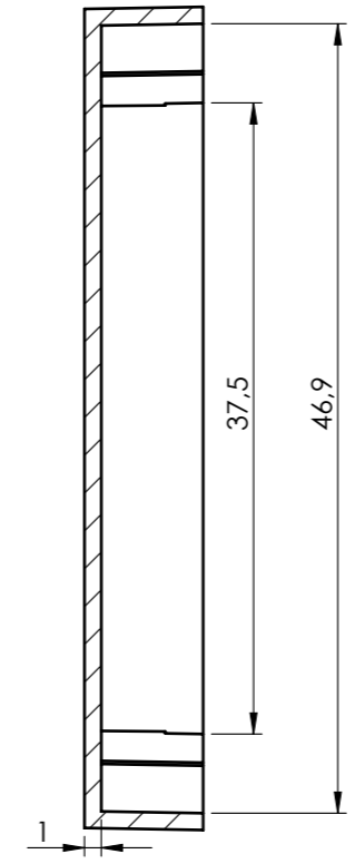
SECTION A-A SCALE 2 : 1
