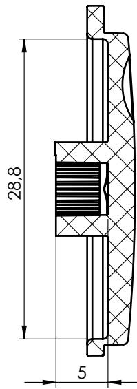
SECTION A-A
